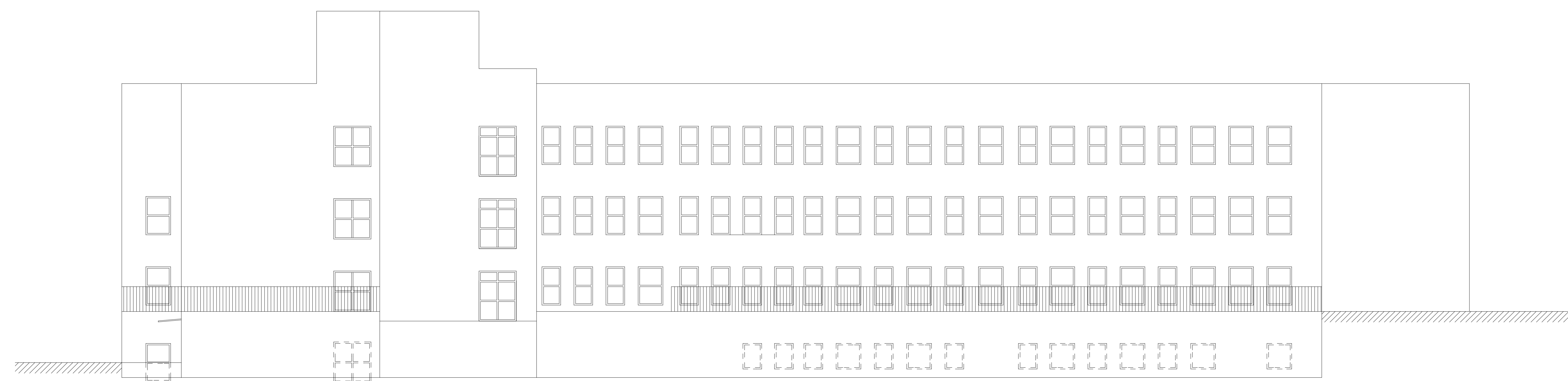
ELEWACJA ZACHODNIA SKALA 1:100
